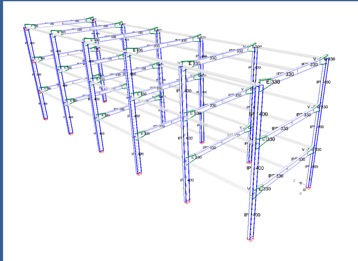
Esquema con SISMO
