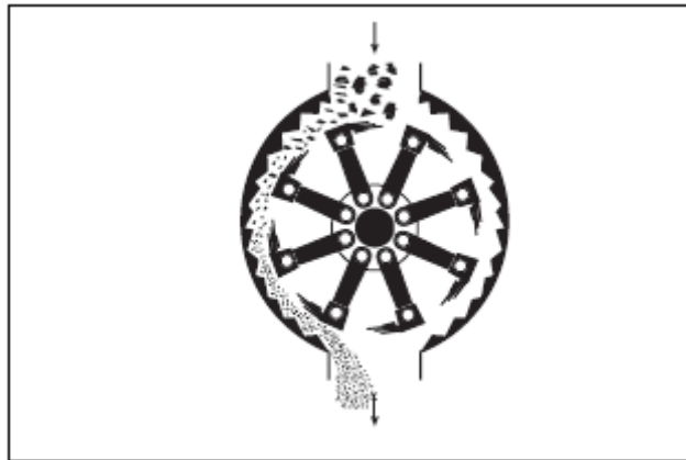
Molino de carbón
