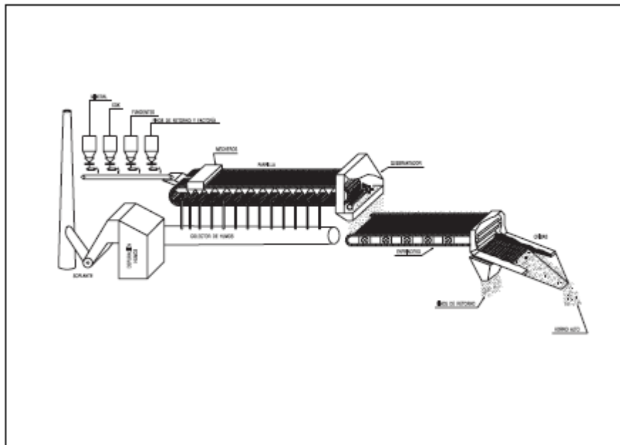
Máquina de sinterizar
