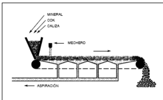
Proceso de sinterización
